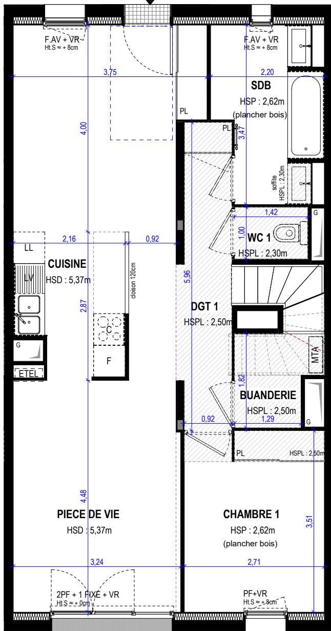
NIVEAU R+1
